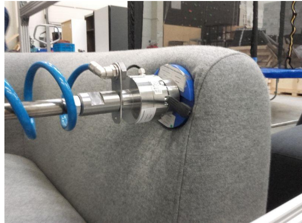
Fotografia / Photo 8 Mechanical testing
