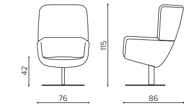
AA 909P LOUNGE high backrest, steel base plate schienale alto, base piastra in acciaio dossier haut, base en tôle d'acier
