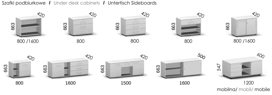
Opcja: zamek szyfrowy Option: Combination lock Option: Zahlencodeschloss
